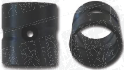
● Sonder AIS mit 1x 10mm Bohrung (mit Außen- und Innenschmierung)
